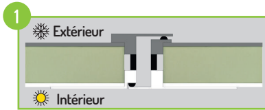
1 Profils à rupture de pont thermique (+ 2 joints EPDM)
